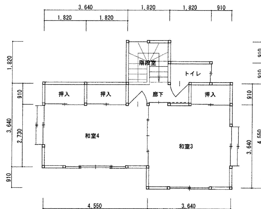
2階平面図 1/100
