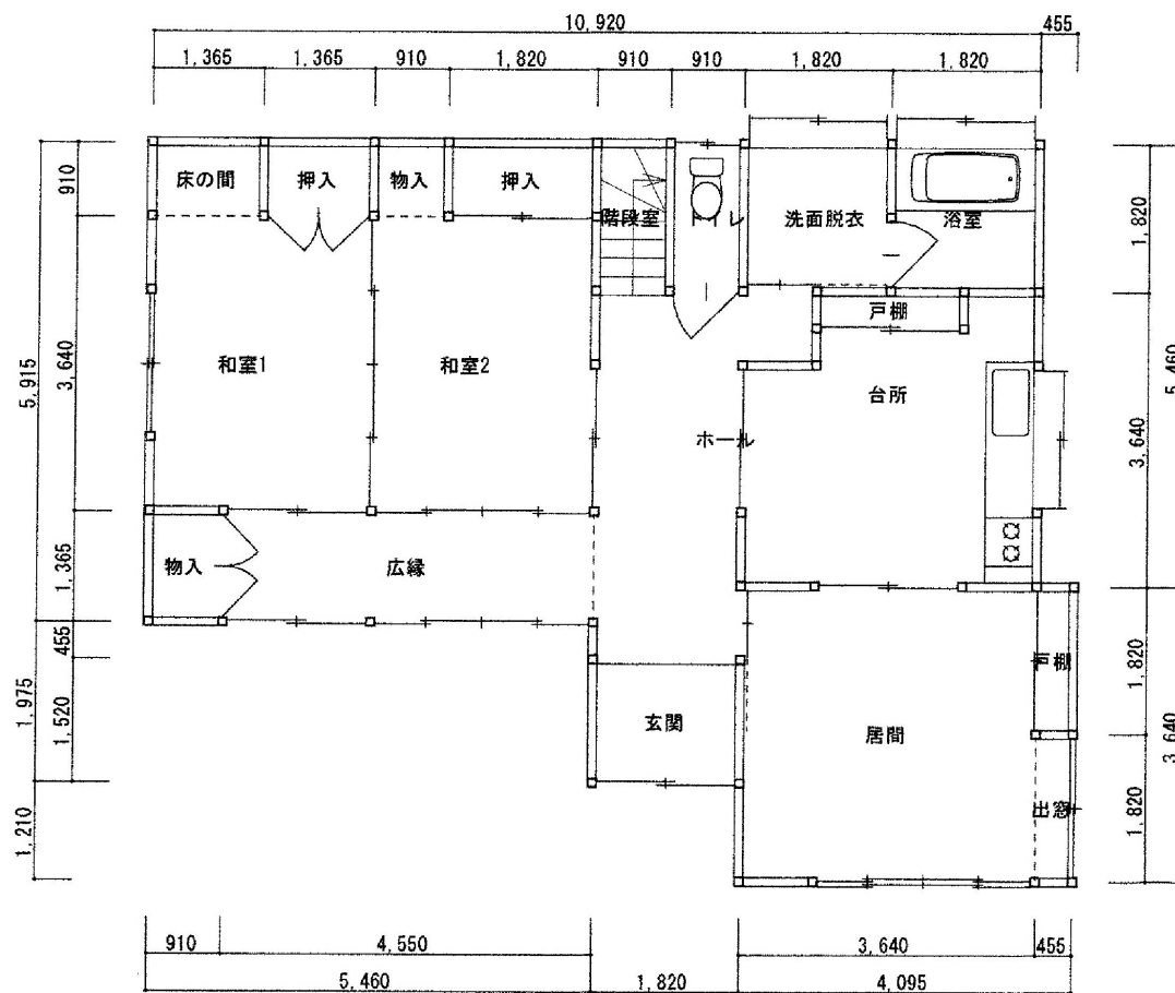
1階平面図 1/100
